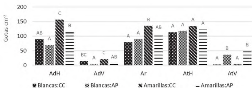
Fig. 2. Densidad de impactos \text{cm}^{-2} contabilizadas por el software Gotas-PC en las diferentes posiciones particionadas por colector tarjetas blancas (papel Glossy) y tarjetas amarillas (papel hidrosensible) y por pastilla AP y CC. Letras diferentes significan diferencias estadísticamente significativas ( p \leq 0.05 ) para el test de Ranks de Kruskal Wallis dentro de cada posición.
