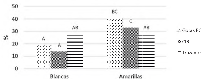
Fig. 4. Comparación de la eficiencia de aplicación cuantificada por los softwares CIR 1.5 y Gotas para pc con dos tipos de colectores, tarjetas blancas (papel Glossy) y tarjetas amarillas (papel hidrosensible) con respecto al trazador colorimétrico. Letras diferentes indican diferencias estadísticamente significativas ( p \leq 0.05 ) para el test de Ranks de Kruskal Wallis.
