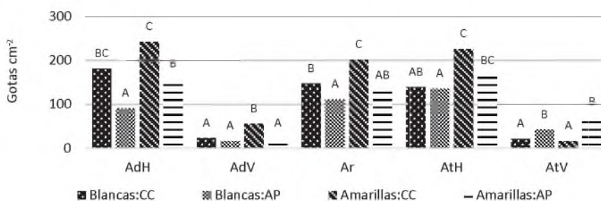
Fig. 3. Densidad de impactos \text{cm}^{-2} contabilizadas por el software CIR 1.5 en las diferentes posiciones particionadas por colector tarjetas blancas (papel Glossy) y tarjetas amarillas (papel hidrosensible) y por pastille AP y CC. Letras diferentes significan diferencias estadísticamente significativas ( p \leq 0.05 ) para el test de Ranks de Kruskal Wallis dentro de cada posición.
